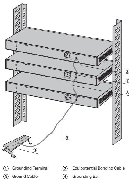
Figure 3-3 Equipotential Bonding
