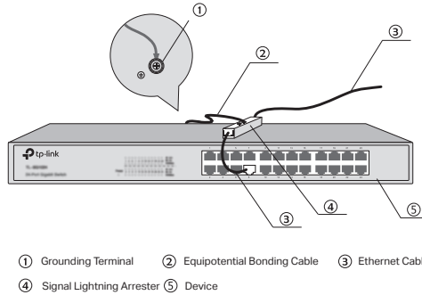
Figure 3-4 Equipotential Bonding
